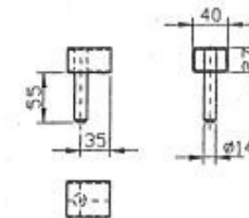
Wspornik siedzenia - 6szt
