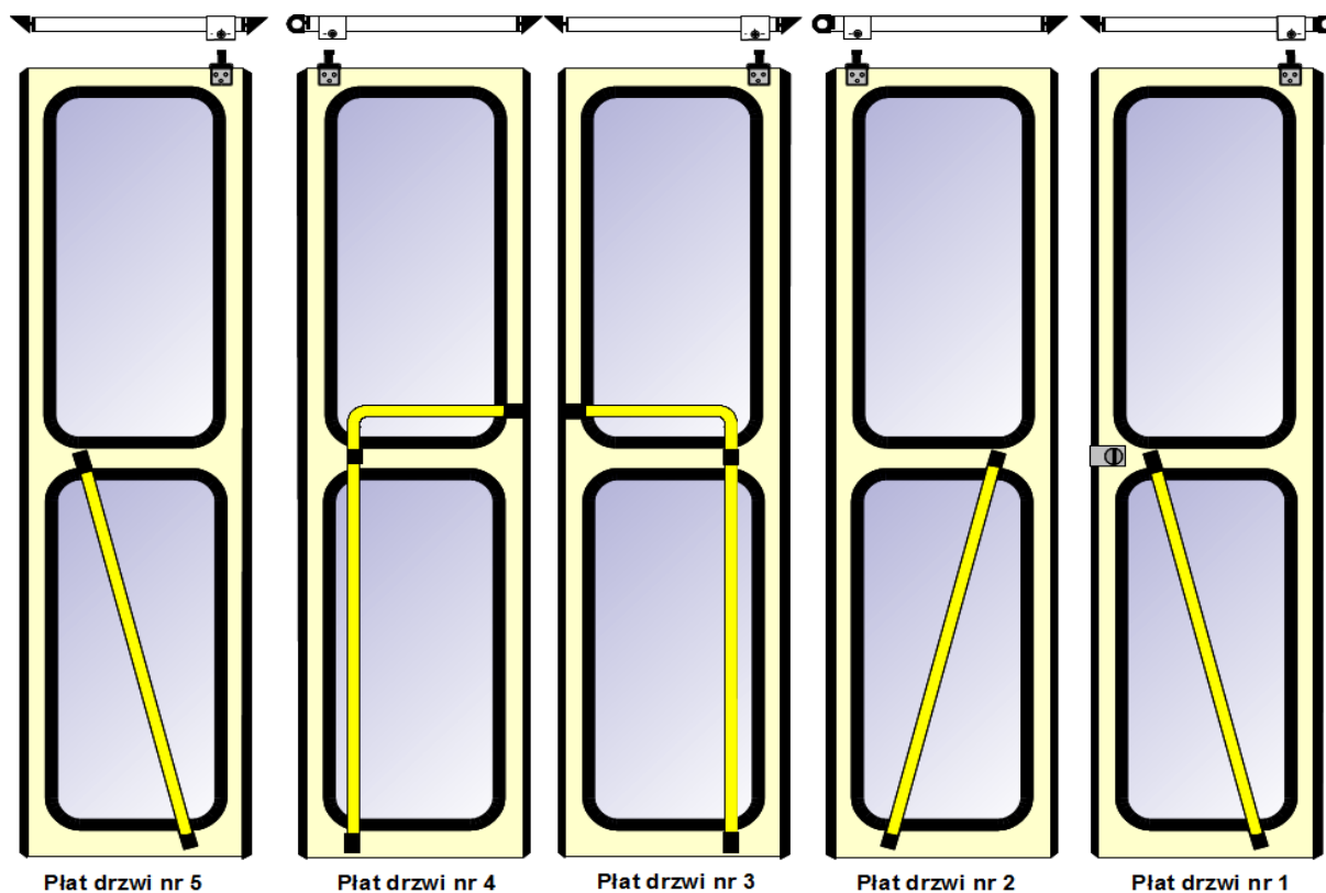
Rysunek nr 2/105Na. Płaty drzwi do wagonu tramwajowego typu 105Na z układem skierowania uszczelek brzegowych – rewers + widok z góry.
