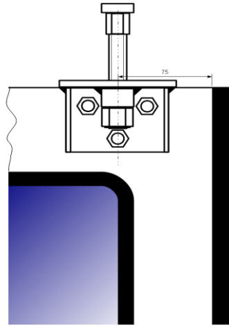
Rysunek nr 7. Zgarniacz miotełkowy drzwi.
