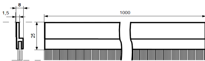
Rysunek nr 7. Zgarniacz miotłkowy drzwi.
