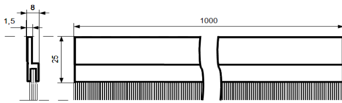
Rysunek nr 7. Zgarniacz miotełkowy drzwi.
