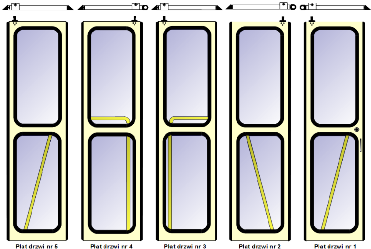
Rysunek nr 1/105Na. Płaty drzwi do wagonu tramwajowego typu 105Na z układem skierowania uszczelek brzegowych – awers + widok z góry.
