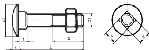
Wymiary dla 3 sztuk śrub zamkowych mocowania wspornika przewodnika drzwi
