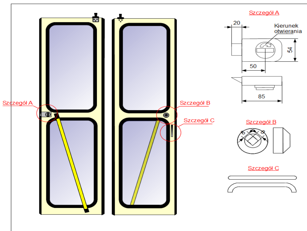
Rysunek nr 3. Płyta drzwi nr 1 w szczegółach.
