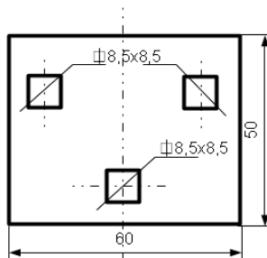
Stalowa blacha oporowa gr. 3 mm mocowania wspornika przewodnika drzwi.
