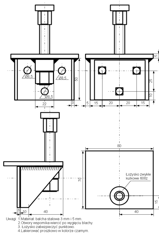
Rysunek nr 8. Usytuowanie przewodnika górnego na płacie drzwi.
