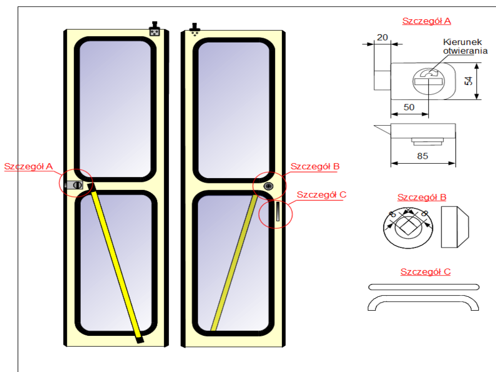
Rysunek nr 3. Płat drzwi nr 1 w szczegółach.
