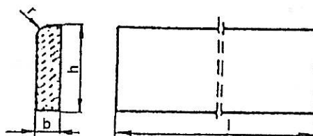
Rysunek 1. Kształt kamiennego obrzeża chodnikowego
