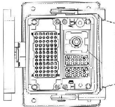
Gniazdo - widok od przodu
