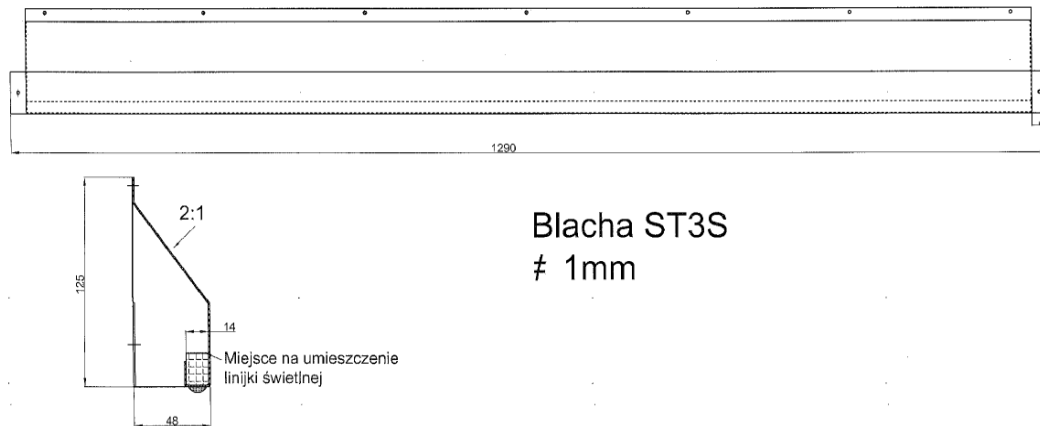
Rysunek nr 3. Listwa doświetlenia strefy przed drzwiami.
