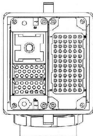
Wtyk - widok od przodu
