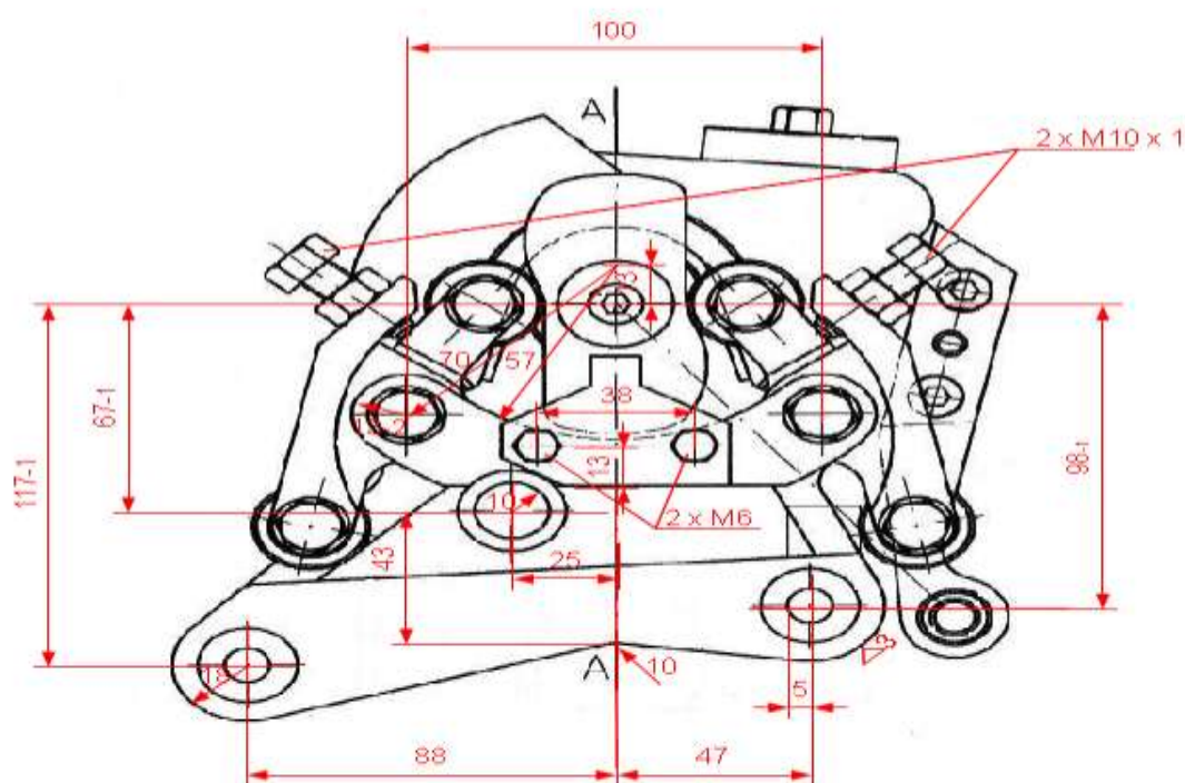
Mechanizm hamulca szczękowego z samoregulatorem – widok od przodu.
