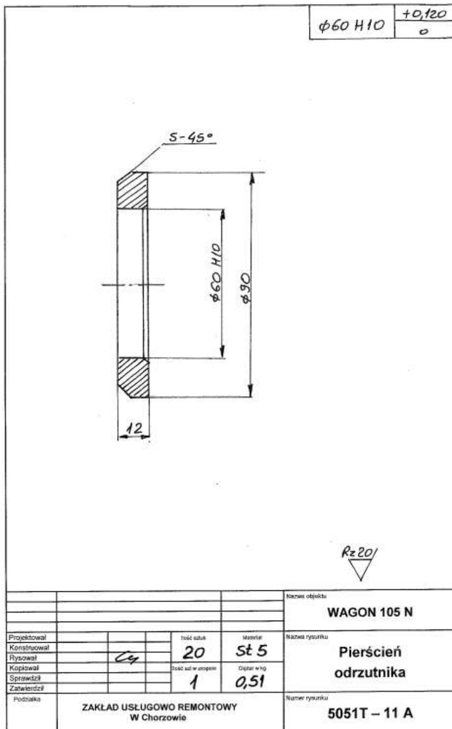
Rys. nr 27 Pierścień odrzutnika oleju do przekładni PM20.
