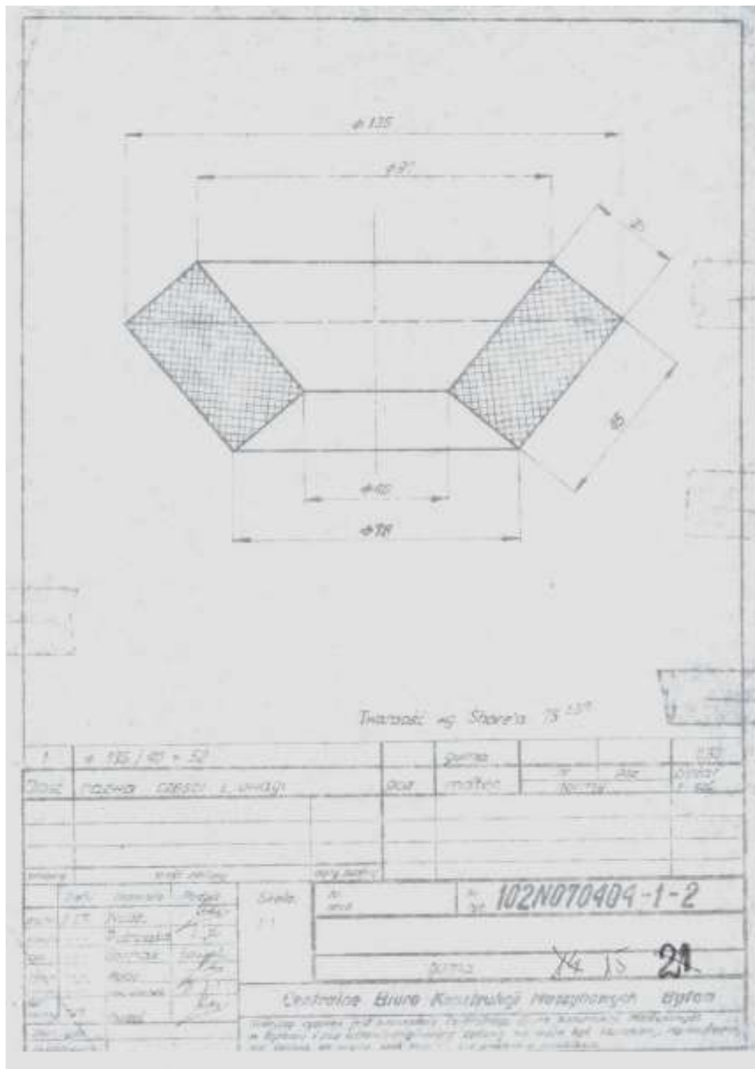
Rys. nr 51 WKŁADKA GUMOWA – wspornik amortyzatora (miseczka)
