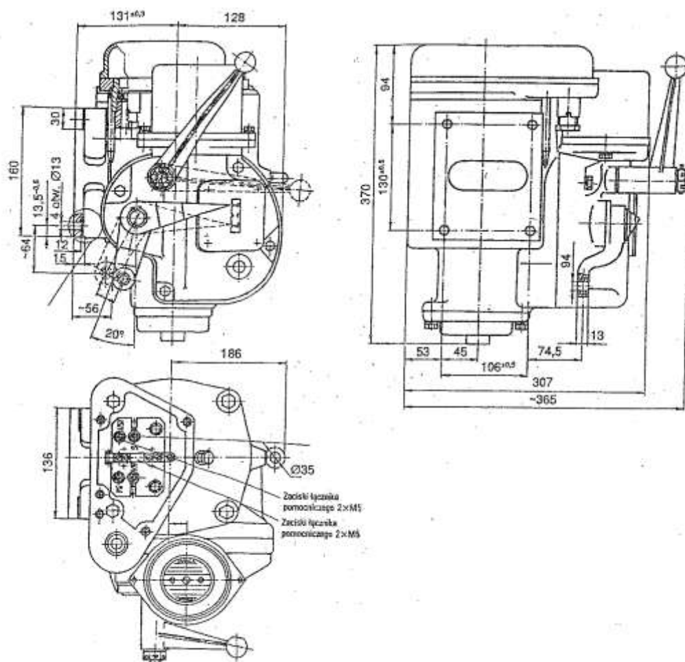
Rys. nr 1 Zwalniak elektromagnetyczny ( luzownik HT – 4).
