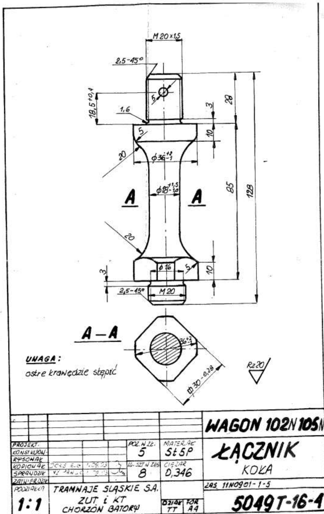
Rys . nr 9 Łącznik koła biegowego
