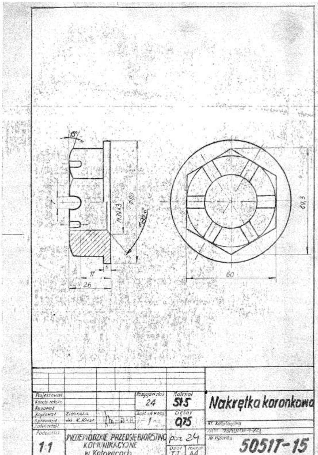
Rys. nr 25 Nakrętka koronkowa przekładni PM20.
