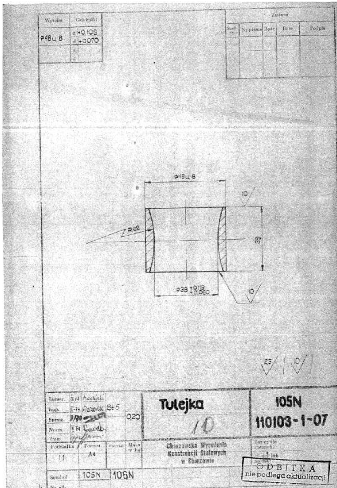
Rys. nr 5 Tulejka.
