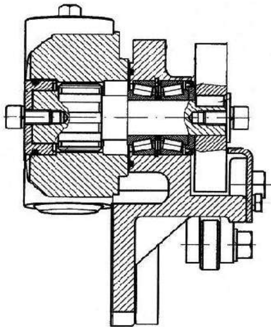
Mechanizm hamulca szczękowego z samoregulatorem - przekrój
