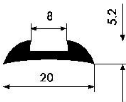
Rysunek nr 1. Profil specjalny – aluminiowy
