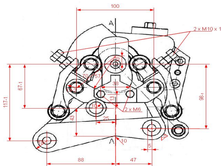
Mechanizm hamulca szczękowego z samoregulatorem – widok od przodu.
