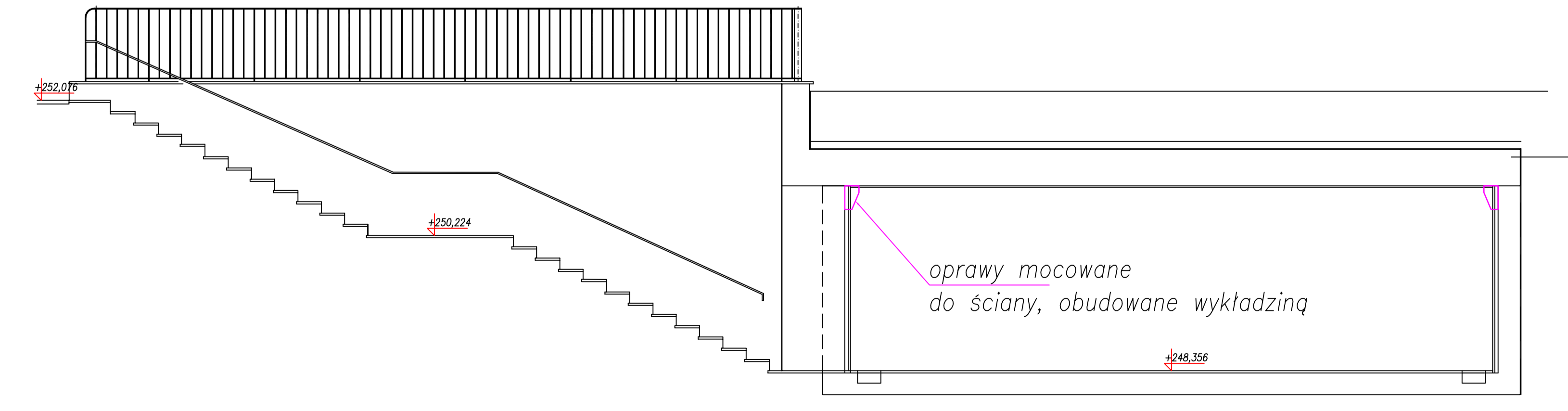
PRZEKRÓJ B - B 1:50
