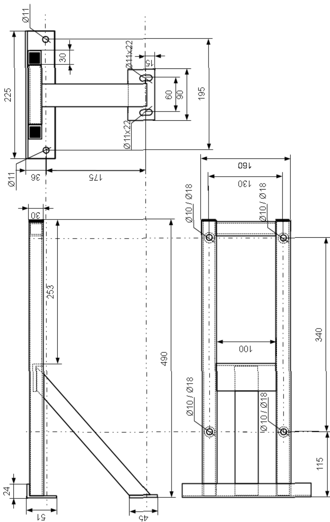
Podstawowe wymiary wspornika dla siedzenia pasażerskiego montowanego do podłogi i do ściany bocznej wagonu 105N
