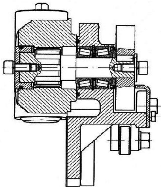
Mechanizm hamulca szczękowego z samoregulatorem - przekrój
