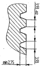
Rozminięcie wienca zębatego
